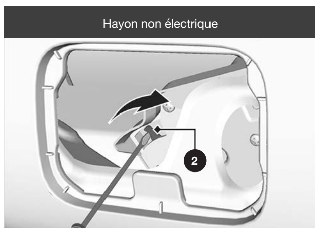
② Levier
