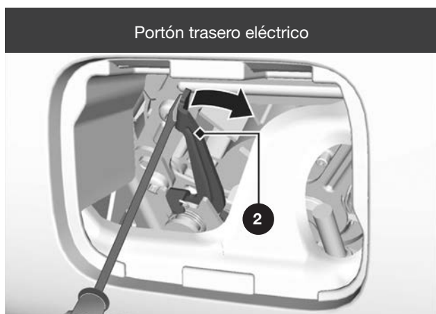
② Palanca
